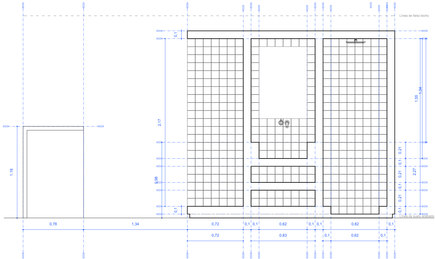
Sección EE'
