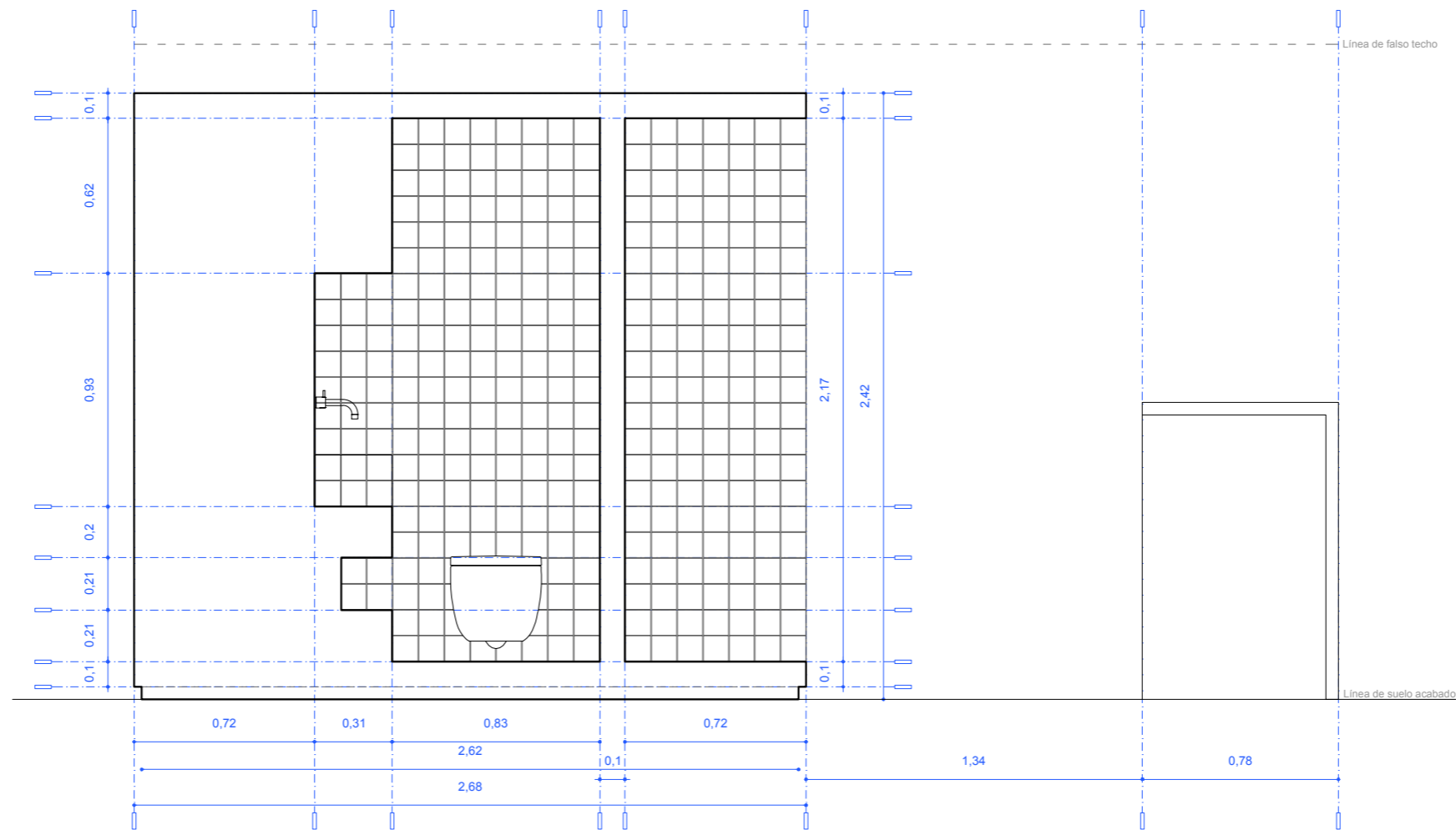
Sección FF'
