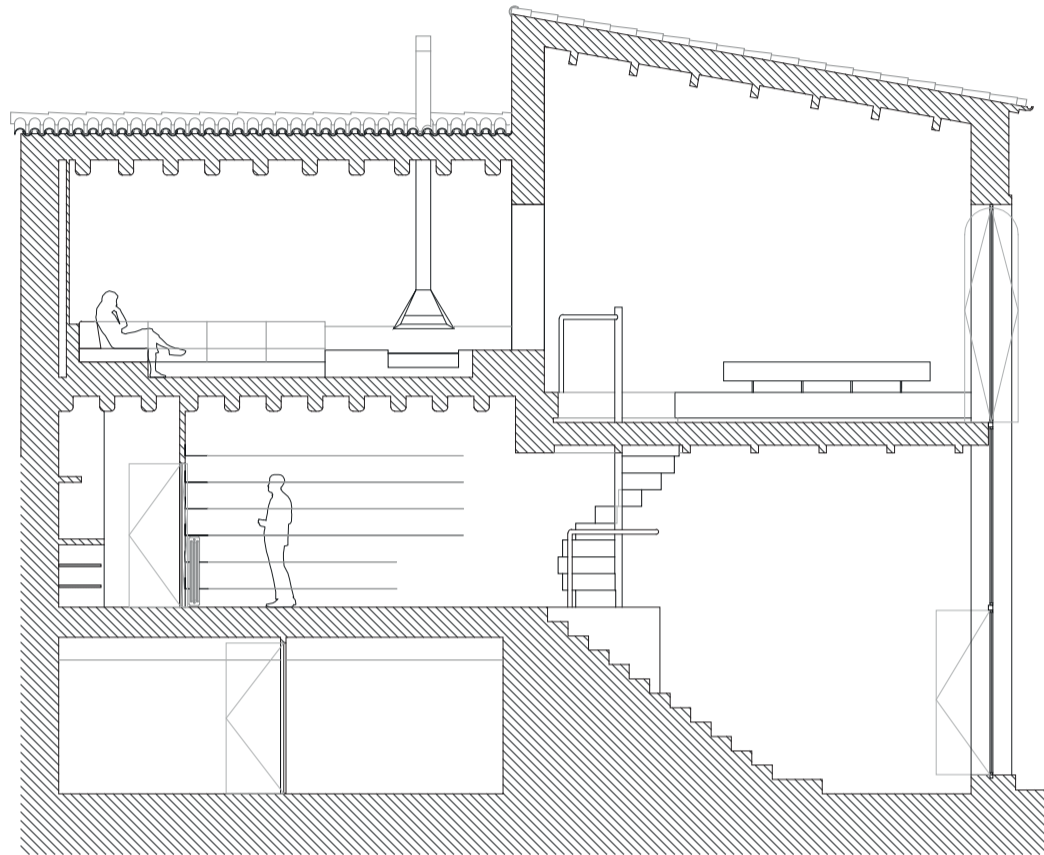
SECCIÓN AA'
