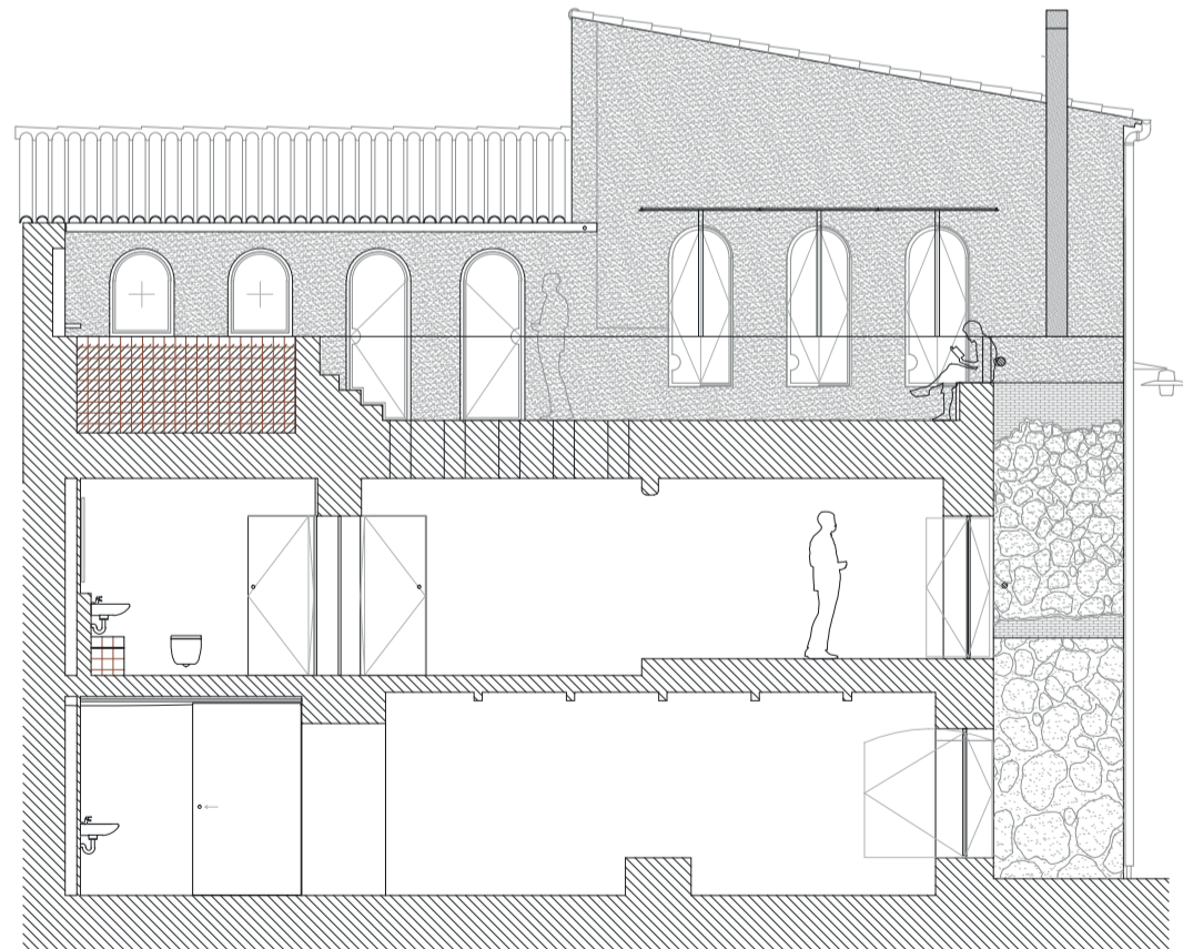
SECCIÓN BB'
